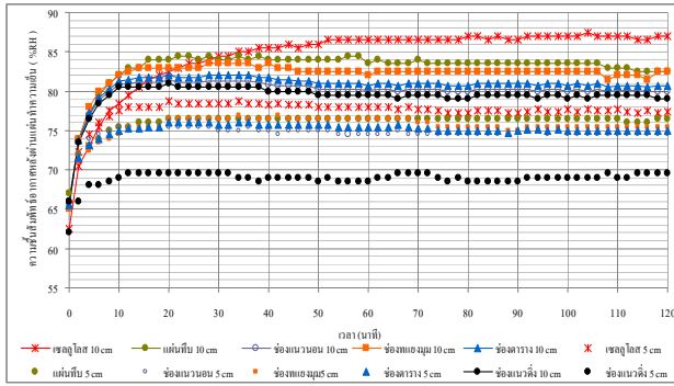
(ก) ความขึ้นอากาศหลังผ่านแผ่นทำความเย็น สภาวะอากาศขาเข้ามีค่า 31 o C
