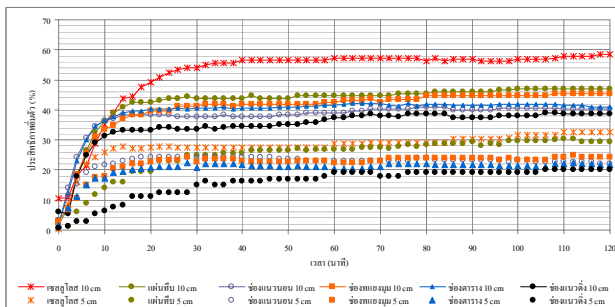
(ก) ประสิทธิภาพอ้อมตัวของแผ่นทำความเย็น สภาวะอากาศขาเข้ามีค่า 31 o C
