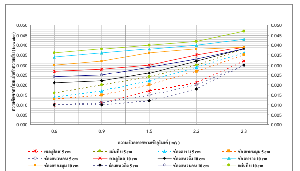
รูปที่ 17 กราฟแสดงความสัมพันธ์ระหว่างความดันตก คร่อมของแผ่นทำความเย็นกับความเร็วกากาศ
