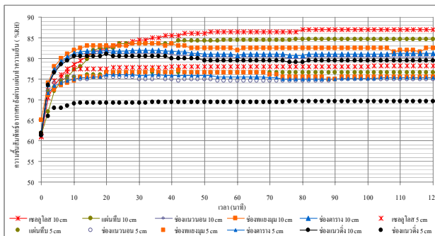
(ข) ความขึ้นอากาศหลังผ่านแผ่นทำความเย็น สภาวะอากาศขาเข้ามีค่า 35 o C
