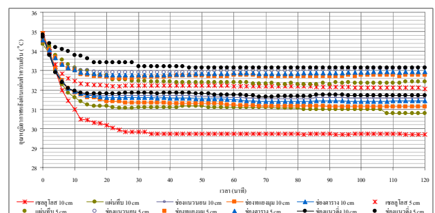
(ข) อุณหภูมิอากาศหลังผ่านแผ่นทำความเย็น สภาวะอากาศขาเข้ามีค่า 35 °C
