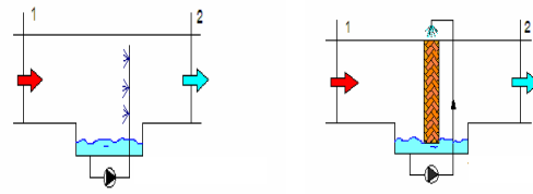
(ก)การพ่นน้ำผ่านอากาศ (ข)การพ่นน้ำผ่านผิวเปียก รูปที่ 1 ภาพการทำความเย็นแบบระเหย
