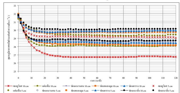
(ก) อุณหภูมิอากาศหลังผ่านแผ่นทำความเย็น สภาวะอากาศขาเข้ามีค่า 31 °C
