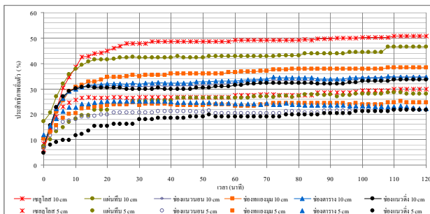
(ข) ประสิทธิภาพอ้อมตัวของแผ่นทำความเย็น สภาวะอากาศขาเข้ามีค่า 35 o C
