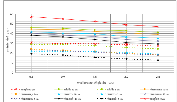
รูปที่ 16 กราฟแสดงความสัมพันธ์ระหว่างประสิทธิภาพ อ้อมตัวของแผ่นทำความเย็นกับความเร็วกากาศ
