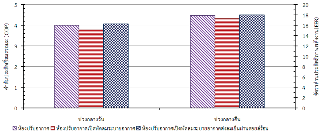
รูปที่ 13 ภาพแสดงการเปรียบเทียบค่า COP และค่า EER ของเครื่องปรับอากาศ
