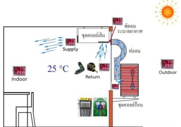
รูปที่ 6 ภาพแสดงห้องปรับอากาศมีการระบายอากาศ
