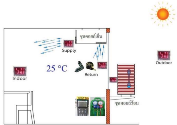
รูปที่ 5 ภาพแสดงห้องปรับอากาศไม่ระบายอากาศ
