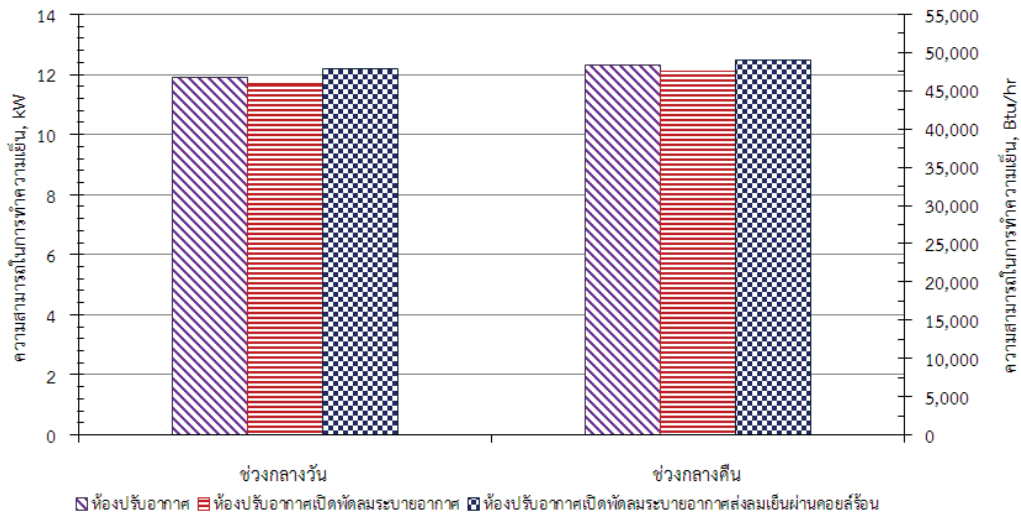
รูปที่ 12 ภาพแสดงการเปรียบเทียบความสามารถในการทำความเย็นของเครื่องปรับอากาศ
