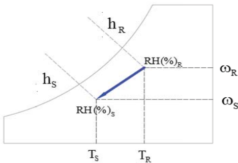
รูปที่ 2 แผนภาพแสดงกระบวนการทำความเย็นและลดความชื้นของเครื่องปรับอากาศบนไฮโครเมตริกชาร์ต
