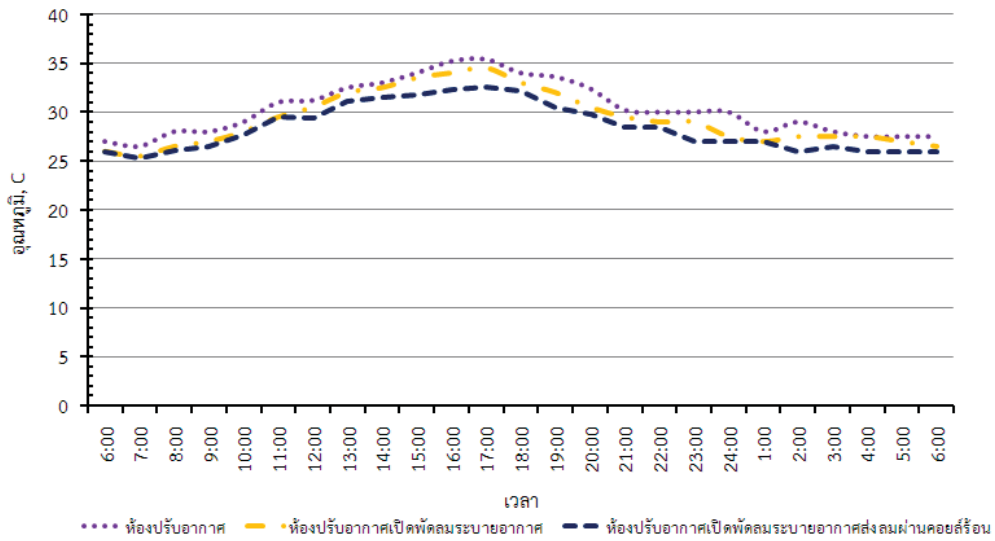
รูปที่ 8 ภาพแสดงการเปรียบเทียบอุณหภูมิอากาศก่อนส่งผ่านชุดคอยล์ร้อน
