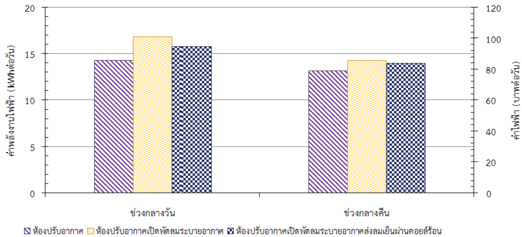
รูปที่ 11 ภาพแสดงการเปรียบเทียบค่าพลังงานไฟฟ้าและค่าไฟฟ้าของเครื่องปรับอากาศ
